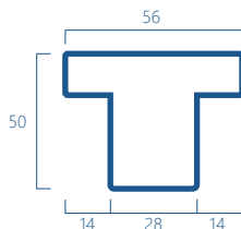
SFG4 Kg/m 2,50
