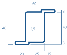
15Z Kg/m 2,45
