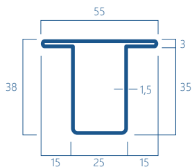
1B Kg/m 2,10
