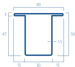
SF2B Kg/m 2.52
