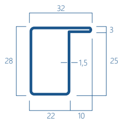
11A Kg/m 1,34
