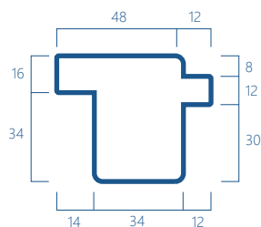
SFG11 Kg/m 2.61
