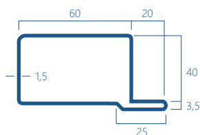
15B Kg/m 2,72
