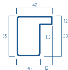
2A Kg/m 1,76
