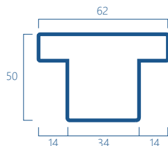
SFG3 Kg/m 2.52
