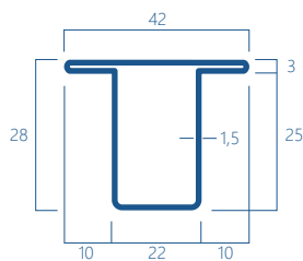
11B Kg/m 1,57
