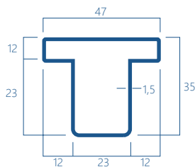
2B Kg/m 1,88
