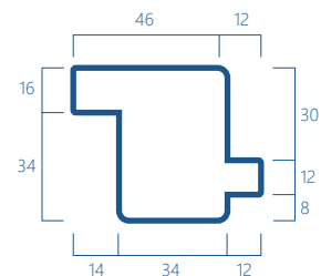
SFG12 Kg/m 2,61
