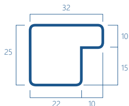
10A Kg/m 1,40
