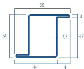
SF3B Kg/m 2.52
