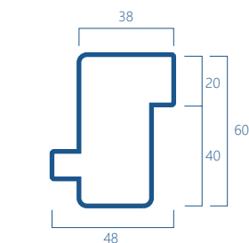
SFG10 Kg/m 2.52
