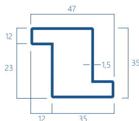
2Z Kg/m 1,88
