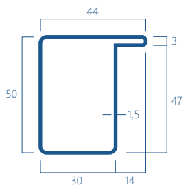
SF1B Kg/m 2.15
