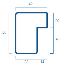
SFG2 Kg/m 2,16
