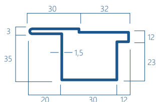
2T Kg/m 2,30
