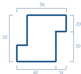
SFG6 Kg/m 2.50
