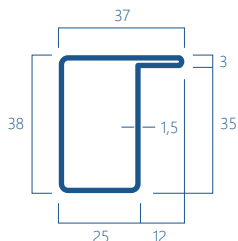
1A Kg/m 1,72
