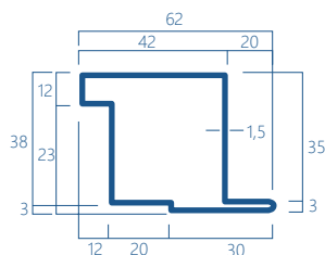
2N Kg/m 2,30
