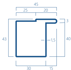
15A Kg/m 2,04
