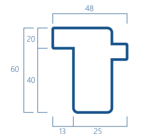
SFG9 Kg/m 2,52
