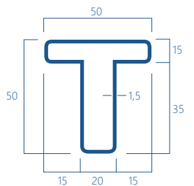
16B Kg/m 2,33
