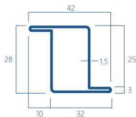
11C Kg/m 1,57
