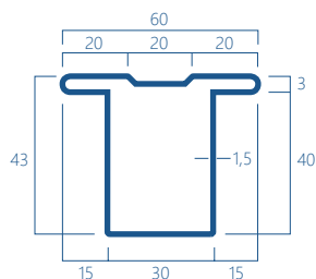
15T Kg/m 2,45
